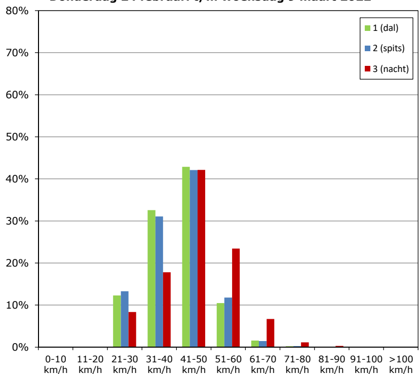
Verdeling snelheden Goirkestraat (ri. zuid) Donderdag 24 februari t/m woensdag 9 maart 2022
