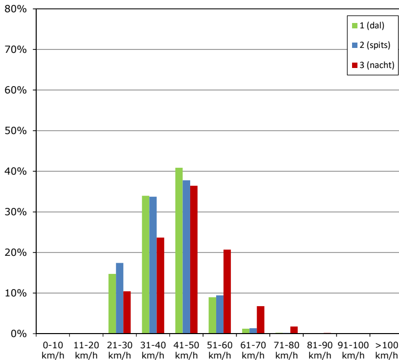
Verdeling snelheden Goirkestraat (ri. zuid) Vrijdag 11 maart t/m donderdag 24 maart 2022
